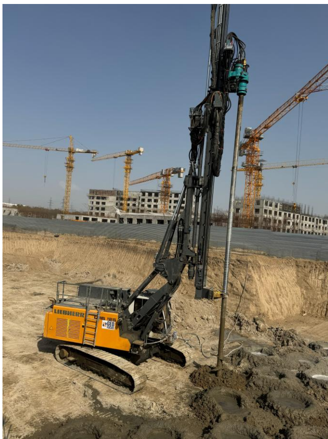
Буровая установка для технологии DSM
